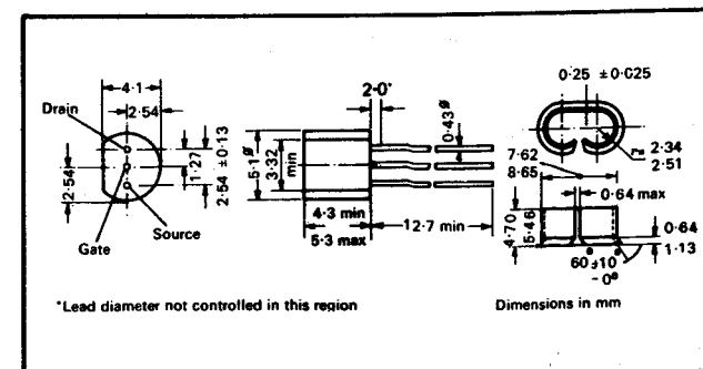
2XTO-92
